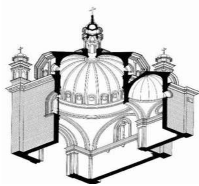
(شكل ٢) قطاع من كنيسة بورتييناري أو القديس بطرس الفيروني الملحقة ببازيليكا سان أوستورجو بميلانو بإيطاليا.
