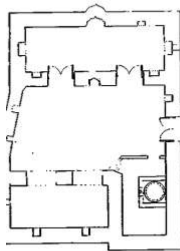
(شكل ١٤) يوضح تخطيط المدرسة العفيفية بمدينة زبيد، عثمان، "المدرسة"، ١٧١.
